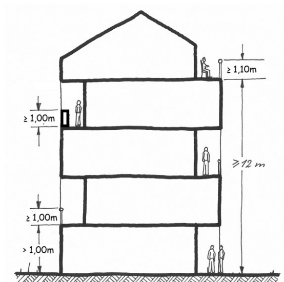
Figure 17 Hauteur des garde-corps
