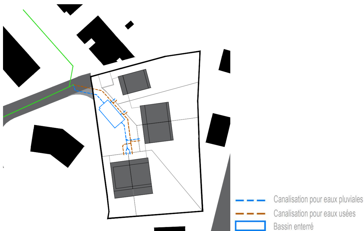
Figure 19 : concept d'assainissement
